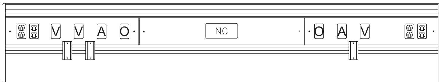
Figure 1. Le module mural de surface de la série «Majestic» avec services sur un niveau
