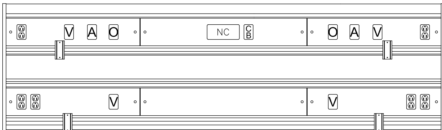
Figure 1. Le module mural de surface de la série «Majestic» avec services sur deux niveaux
